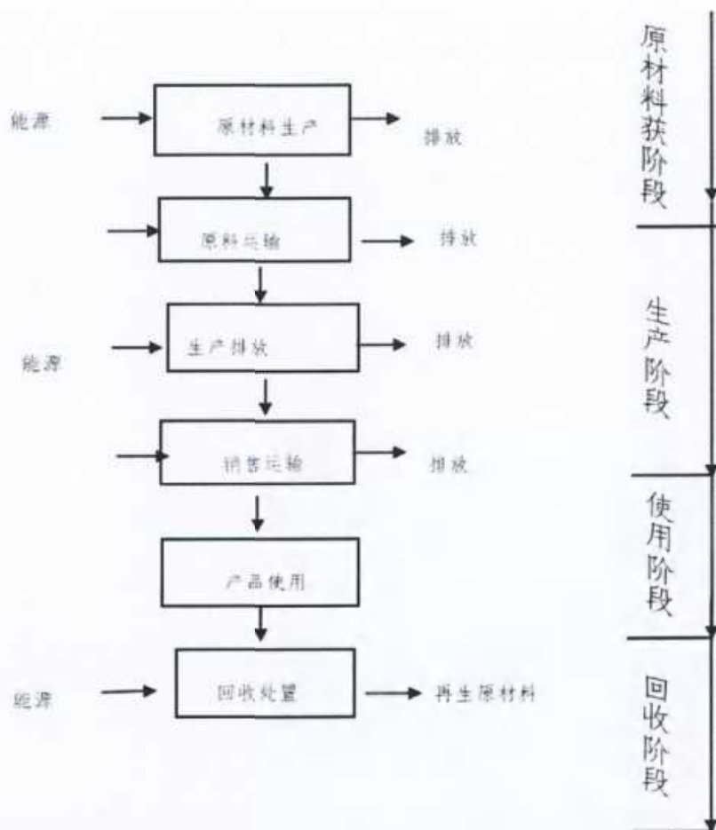
图 1 热缩套管的生命周期系统边界图
